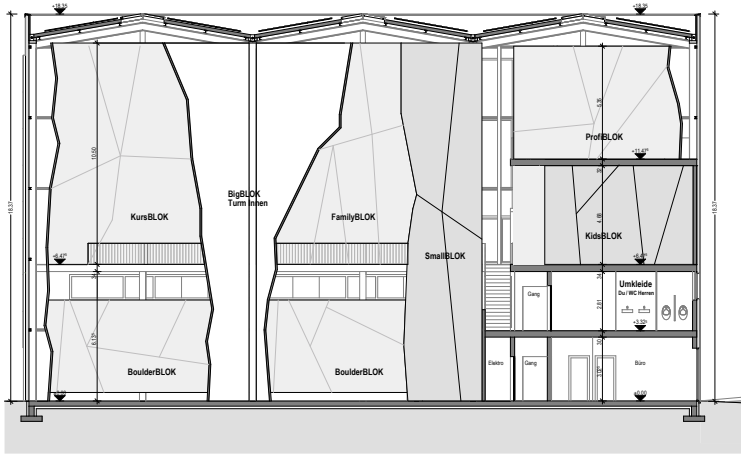
Schnitt 2
