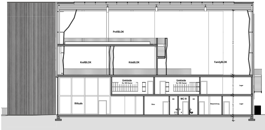
Schnitt 4
