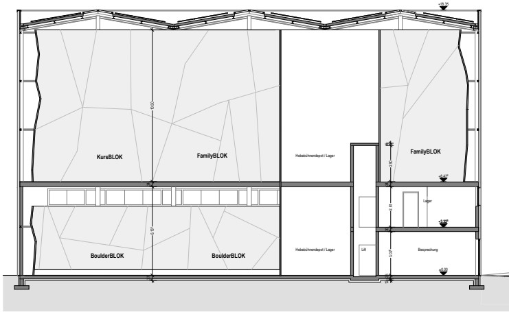
Schnitt 3
