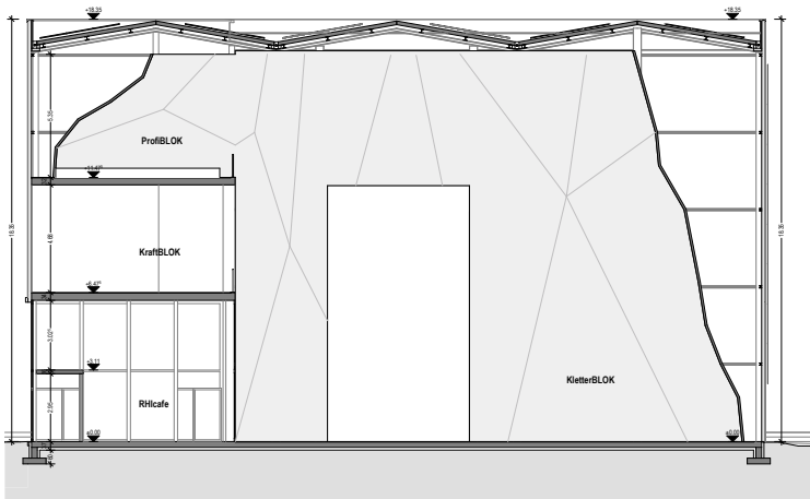
Schnitt 1
