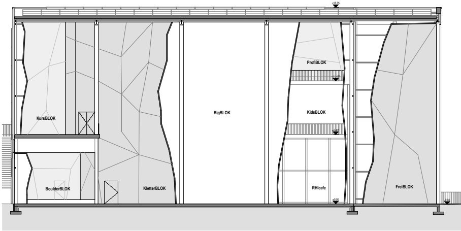
Schnitt 6
