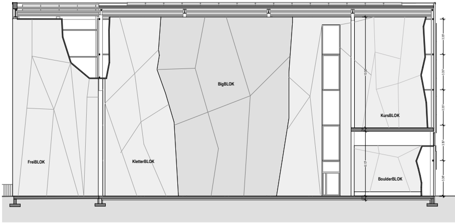
Schnitt 5
